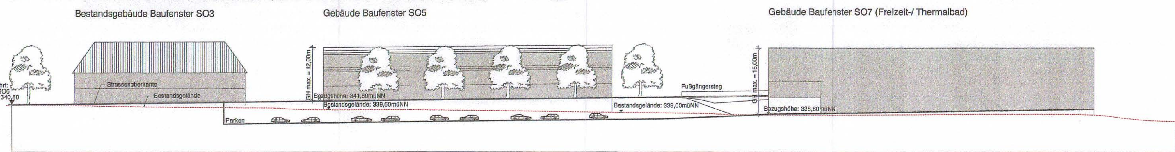
SCHNITT A-A: ANLIEGERSTRASSE (BAUFENSTER SO3/SO5/SO6) M 1:500
